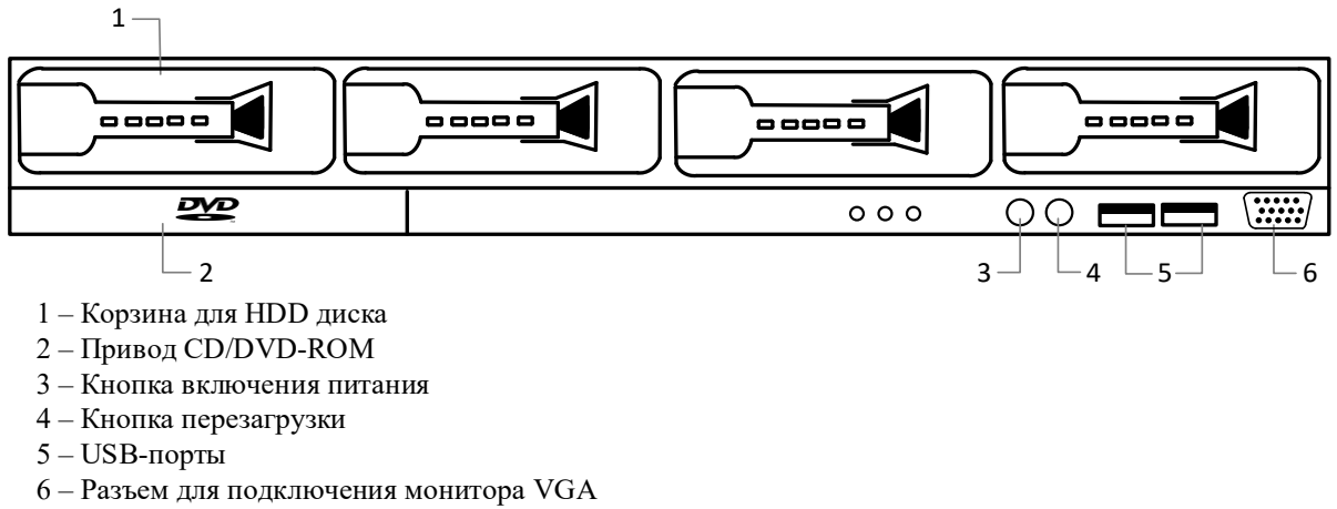
Рисунок 3. Передняя панель прокси-сервера для АПК InfoDiode PRO
