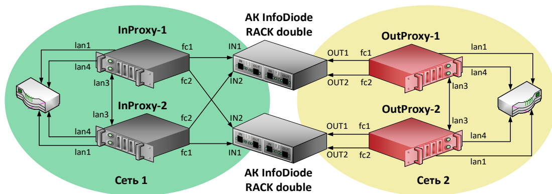
Рисунок 13. Схема подключения кластерной версии АПК InfoDiode PRO cluster к корпоративной сети.
