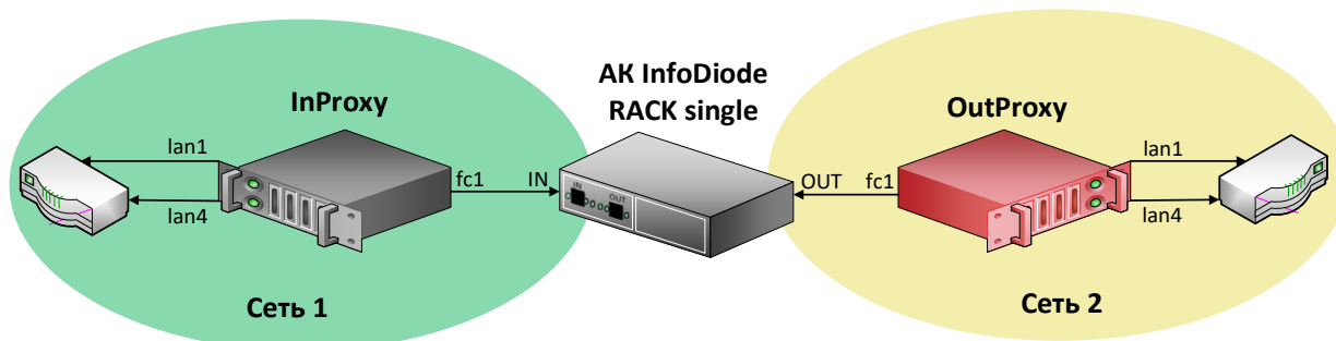
Рисунок 6. Схема подключения АПК InfoDiode PRO base к корпоративной сети.
