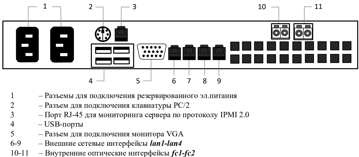
Рисунок 4. Задняя панель прокси-сервера для АПК InfoDiode PRO
