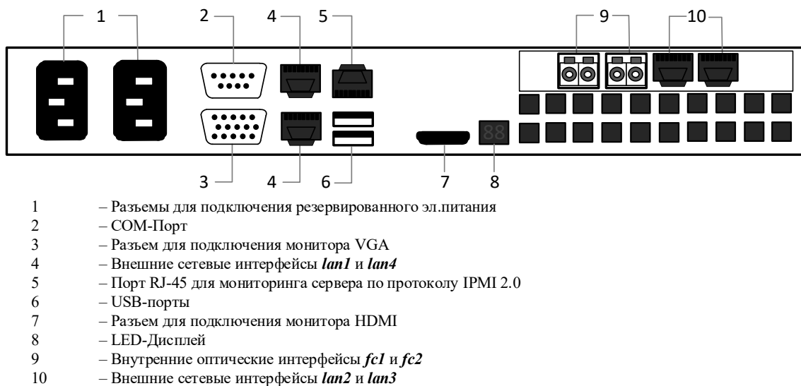
Рисунок 12. Задняя панель прокси-сервера (модель EL108) для АПК InfoDiode PRO
