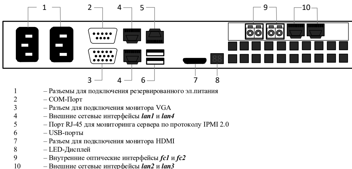
Рисунок 5. Задняя панель прокси-сервера (модель EL108) для АПК InfoDiode PRO
