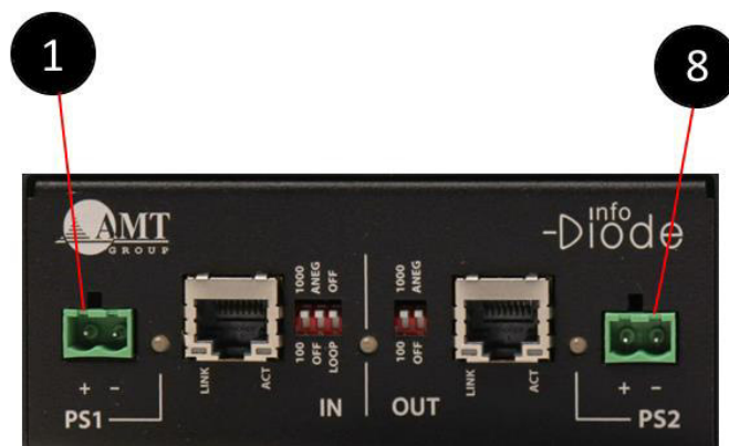
Рис. 7. Разъемы электропитания
