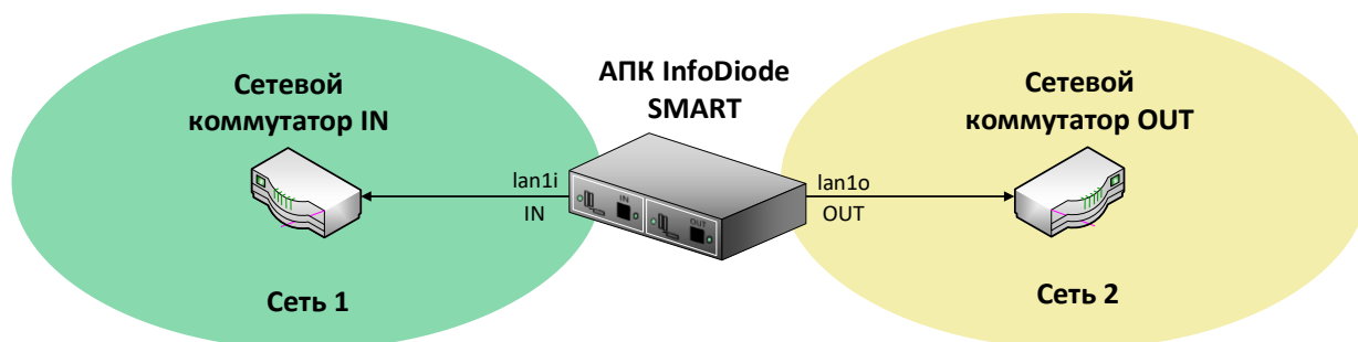
Рисунок 3. Схема подключения АПК InfoDiode SMART к корпоративной сети.
