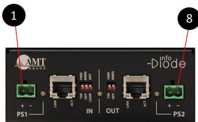
Рис. 7. Разъемы электропитания
