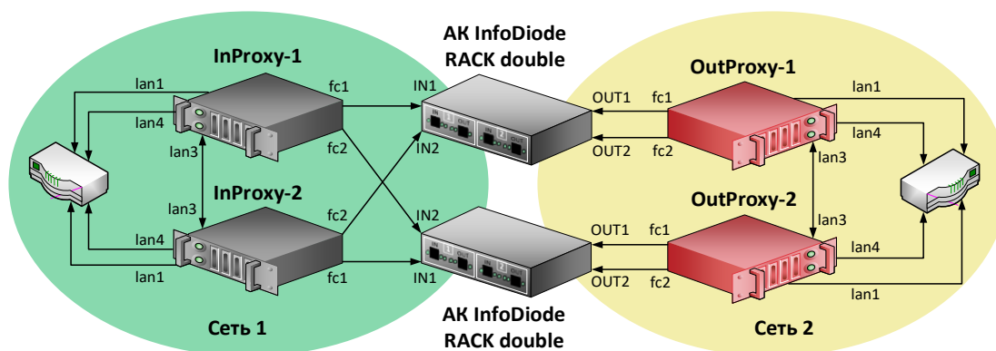
Рисунок 17. Схема подключения кластерной версии АПК InfoDiode PRO cluster к корпоративной сети.
