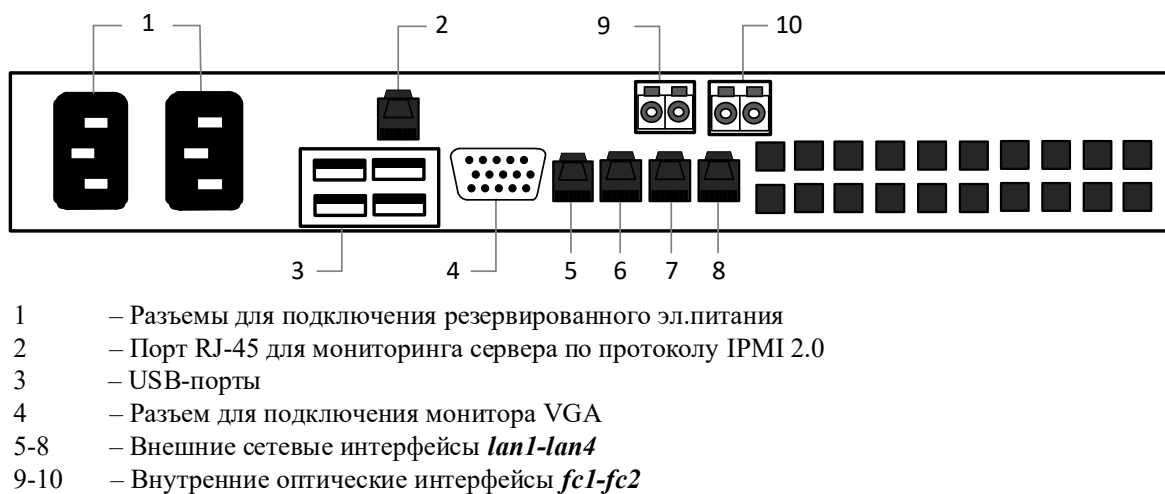
Рисунок 7. Задняя панель прокси-сервера (модель T40 S104DF) для АПК InfoDiode PRO
