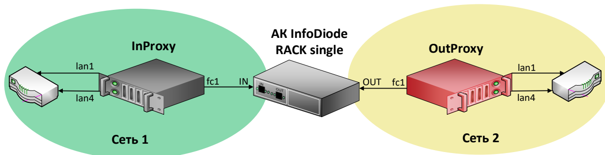
Рисунок 8. Схема подключения АПК InfoDiode PRO base к корпоративной сети.
