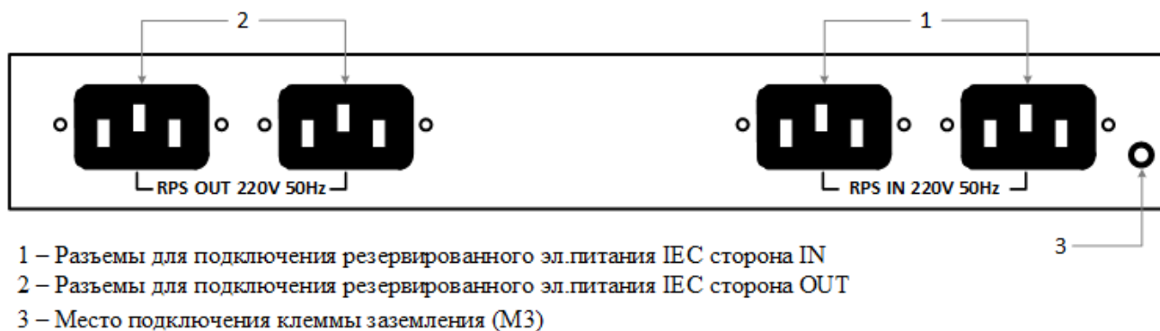
Рисунок 2. Задняя панель устройства однонаправленной передачи данных АПК InfoDiode SMART
