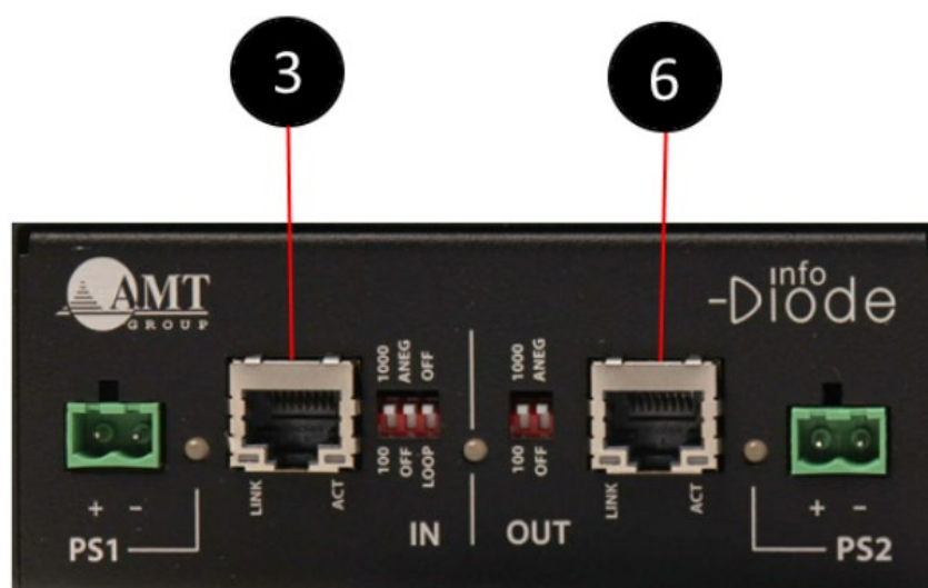
Рис. 9. Разъемы для подключения
