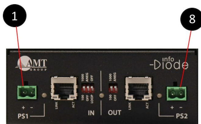
Рис. 7. Разъемы электропитания
