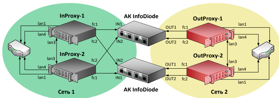
Рисунок 11. Схема подключения кластерной версии АПК «InfoDiode» к корпоративной сети.
